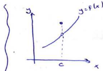
f(x) , c 'de süreksiz. Çünkü \lim_{x \rightarrow c} f(x) \neq f(c) .
